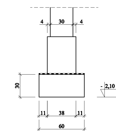
C - C skala 1:25
