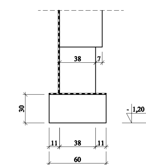
b - b skala 1:25
