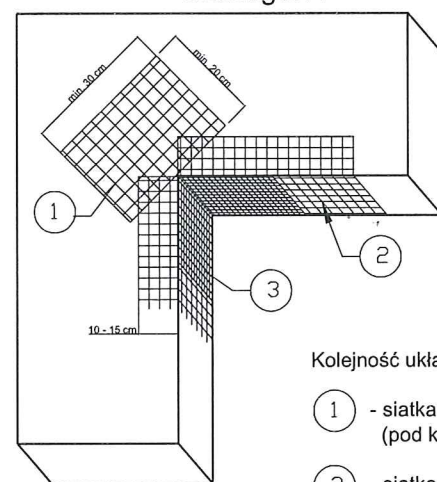
Szczegół A
